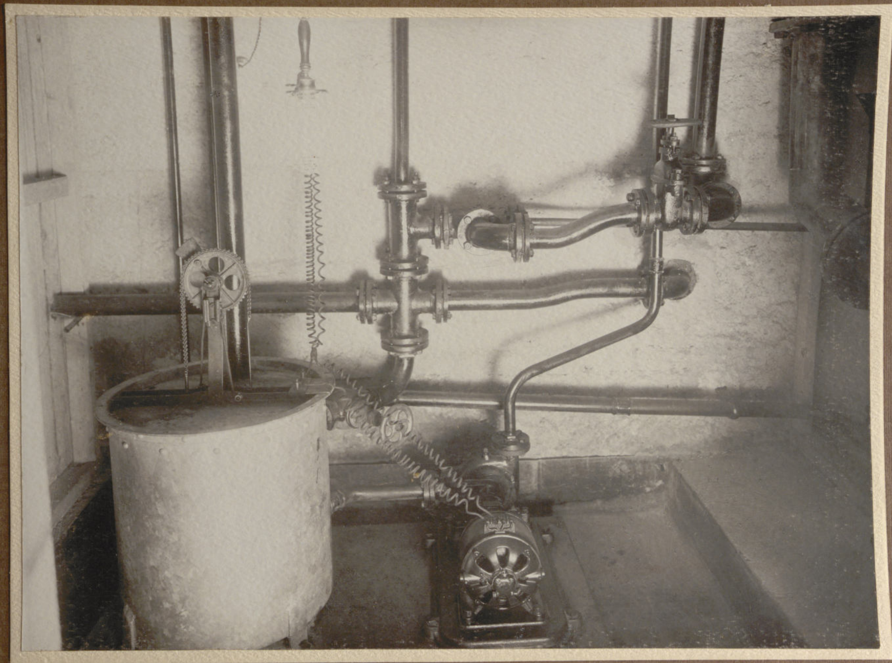
Kondensrückspeise-Anlage,
