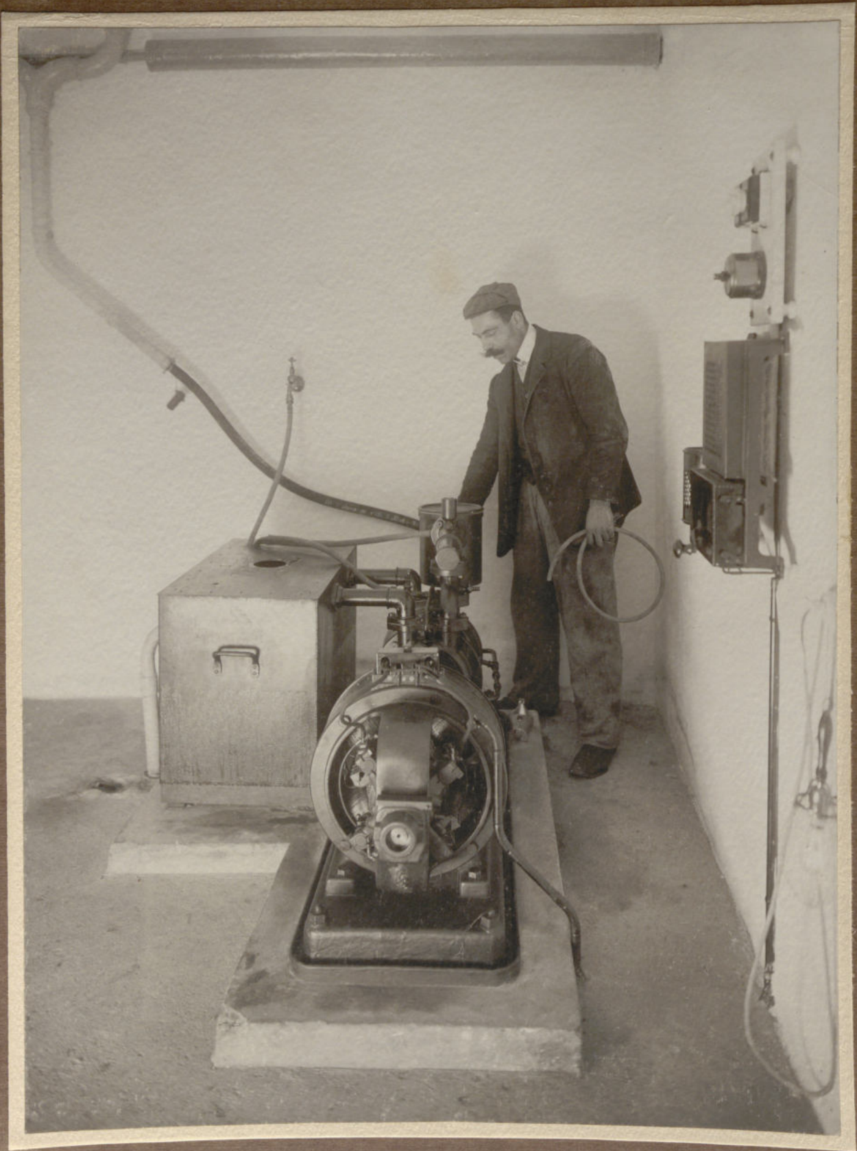
Staubfang-Anlage,
