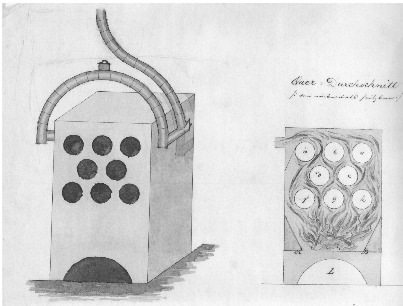
Entwurf einer Zentralheizung für das Schul- und Amtsgebäude der Gemeinde Weikersdorf, Josef Gregora jun.
