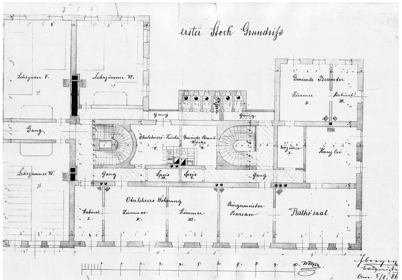
Baupläne für das Schul- und Amtsgebäude der Gemeinde Weikersdorf, Bmst. Franz Breyer, 5./8. 1868 (aus dem Bauplanarchiv der Fa. Baumeister Steurer)
